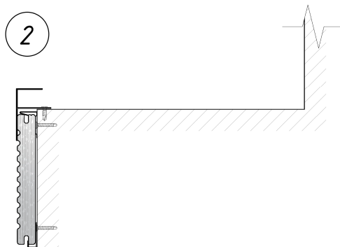
Рис. 7.2. Установка F-профиля
