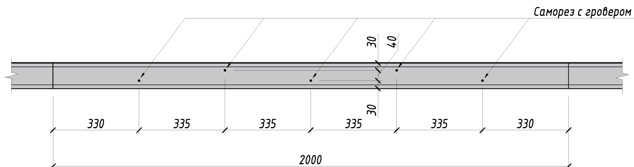
Рисунок 5.11. Вид Б
