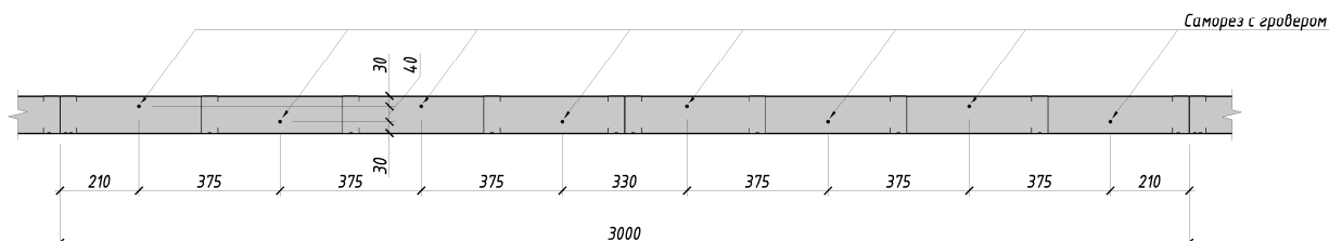
Рисунок 5.10. Вид А
